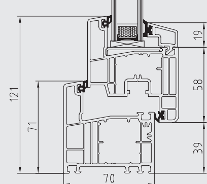
Fenster 1-flügelig, Dreh-Kipp
