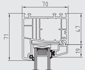
Oberlicht fest
