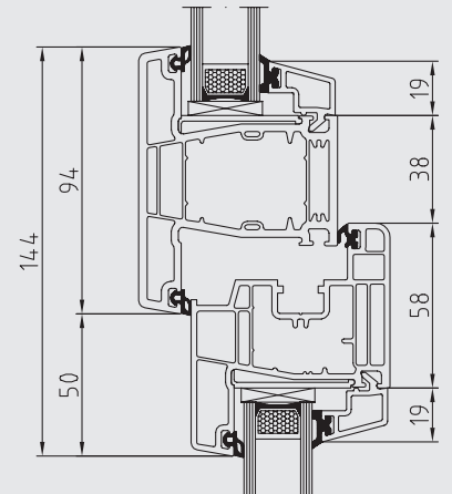
Fenster 1-flügelig, Dreh-Kipp
